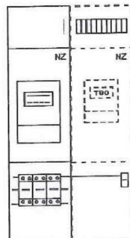
Erweiterung: Sammelschienensystem mit NH-Schalter
