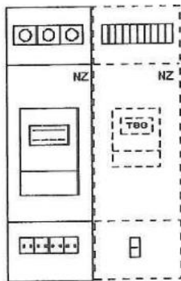
Erweiterung: Anbaukasten mit Klemmstein und Kunden-Hauptsicherung
