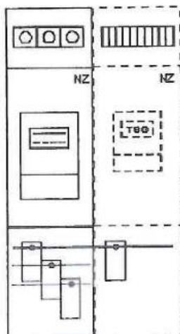
Erweiterung: Sammelschienensystem mit NH-Elementen und Kunden-Hauptsicherung
