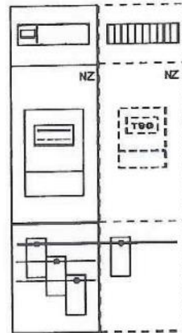
Erweiterung: Sammelschienensystem mit NH-Sicherungen und Kunden-Hauptschalter
